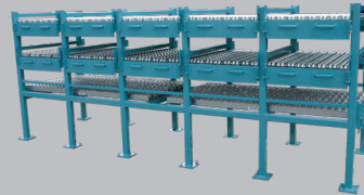
6752 Die Storage Rack
